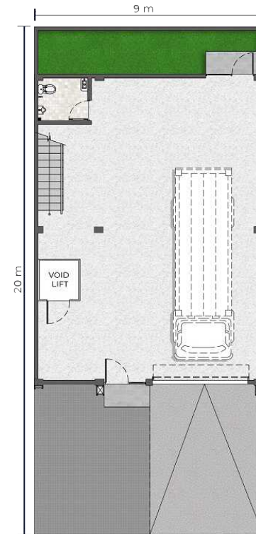
DENAH LT.1
