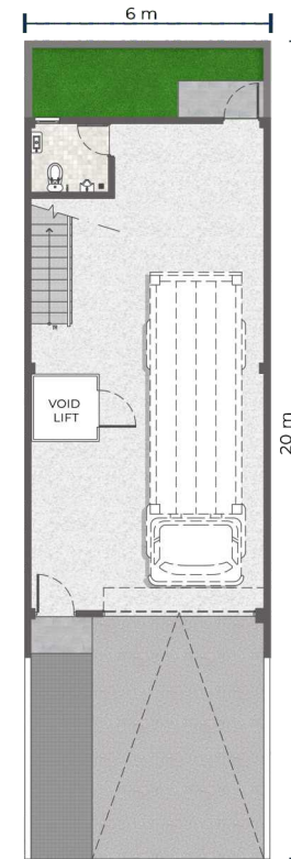
DENAH LT.1
